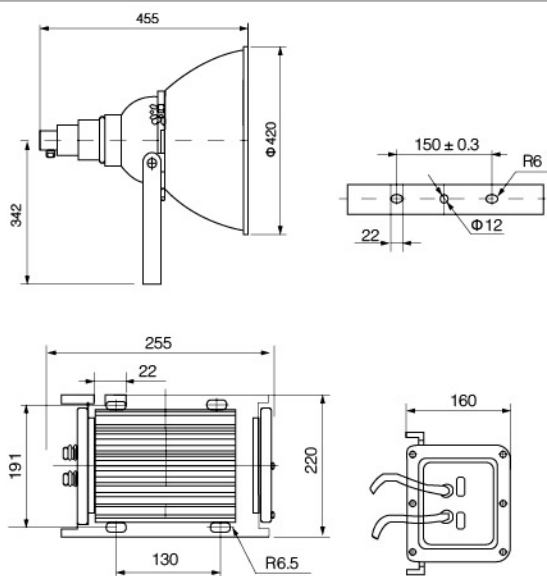
三防镇流器箱
