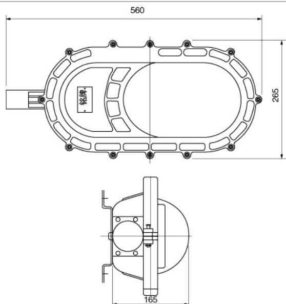
外形尺寸图 External dimensions
