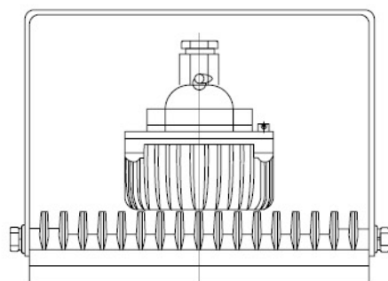
吸顶式 Ceiling type
