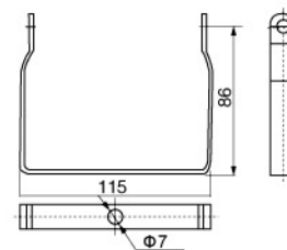
坐式安装附件图
