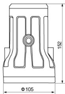
外形图
