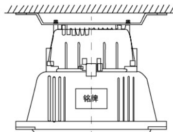
吸顶式 Ceiling type
